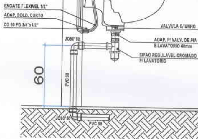
Detalhe Lavatórios Escala: s/ escala
