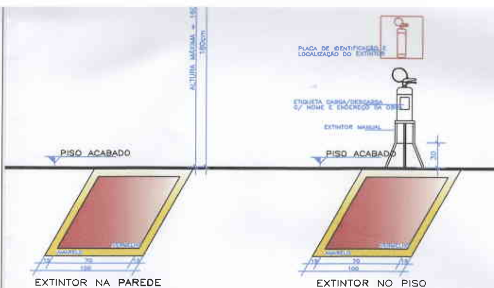
DETALHE: EXTINTOR ESCALA= SEM ESCALA
