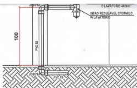
Detalhe Pia Escala: s/ escala
